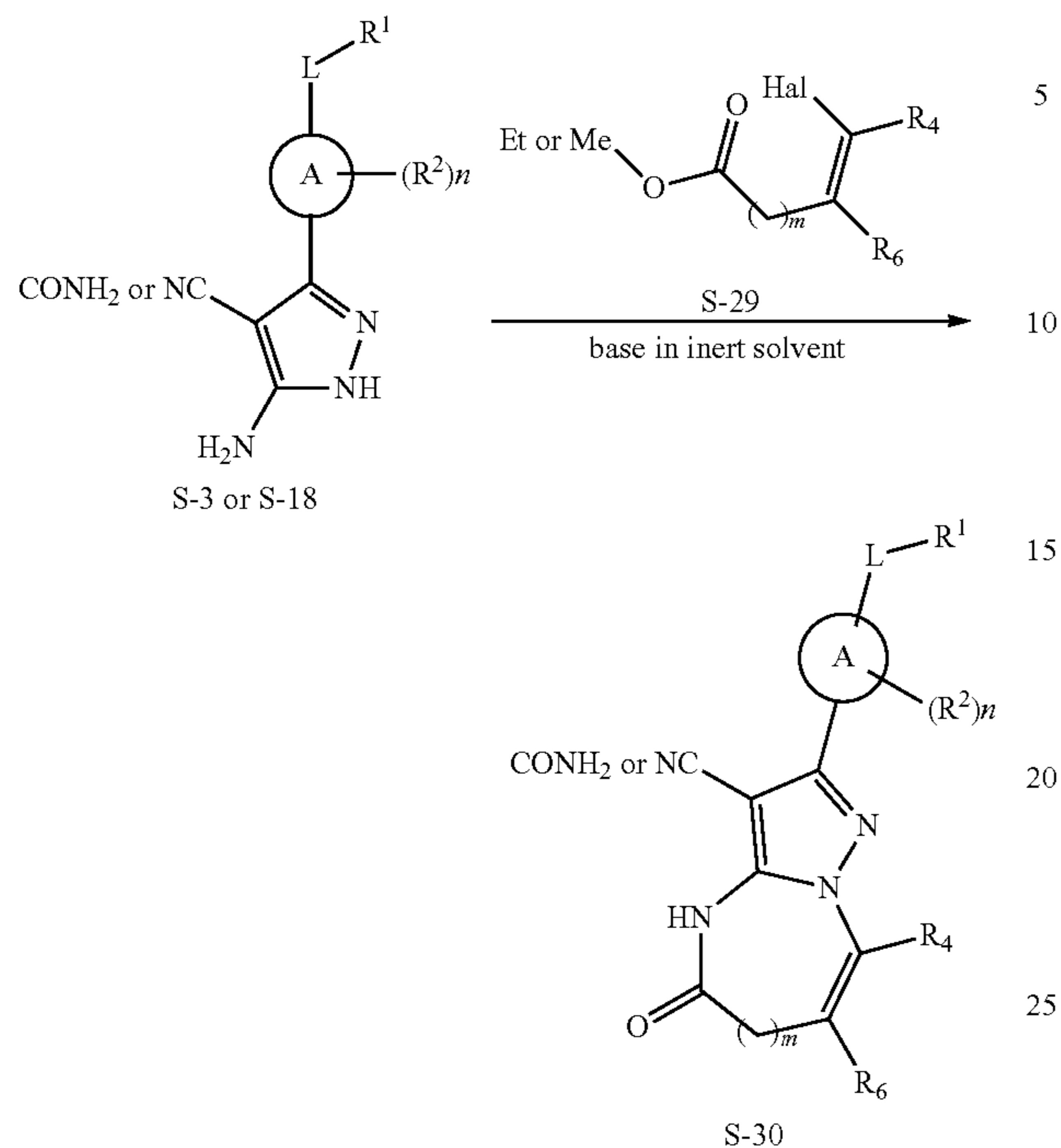
Scheme VI
