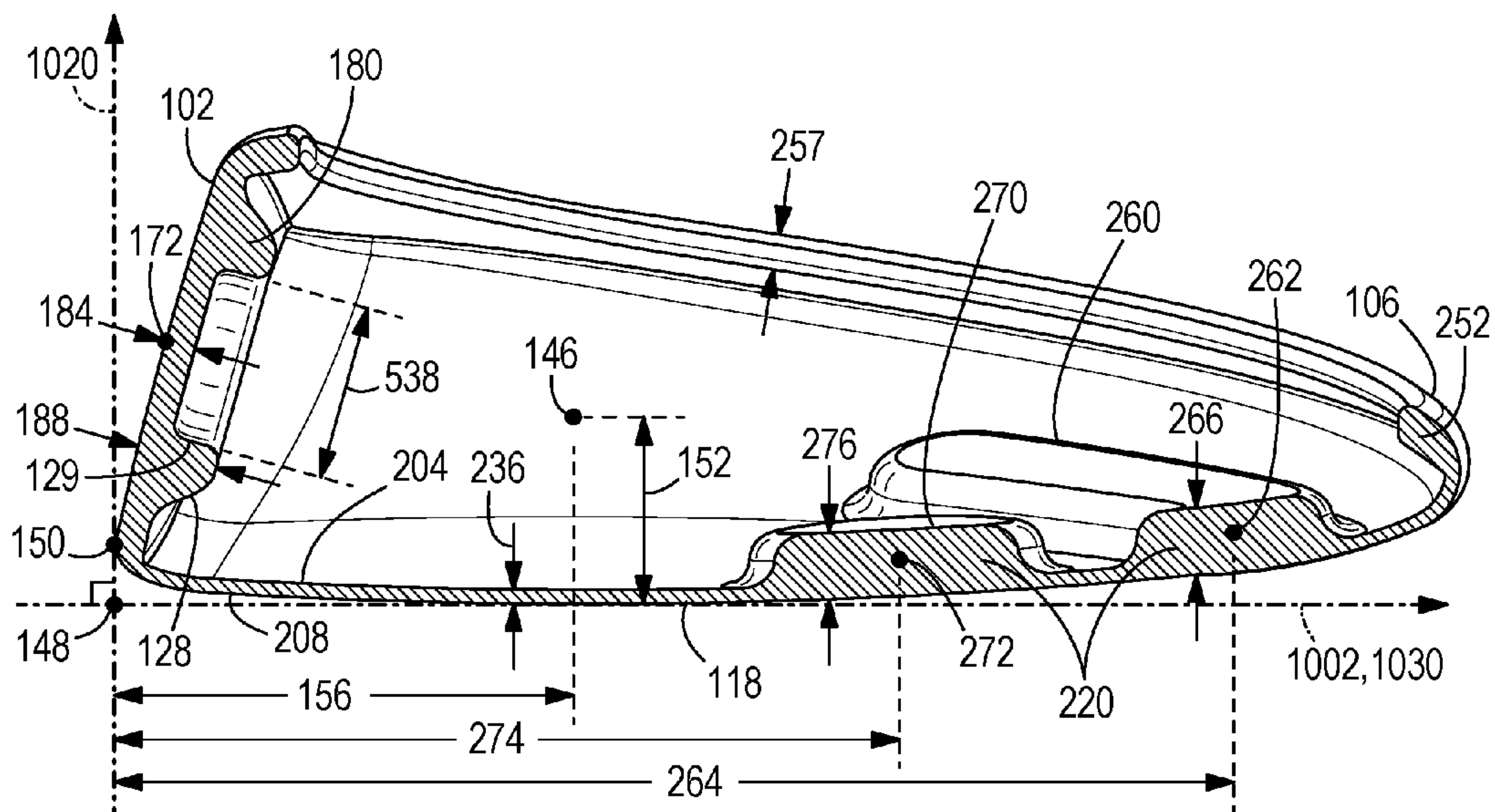
FIG. 6 Section A-A
