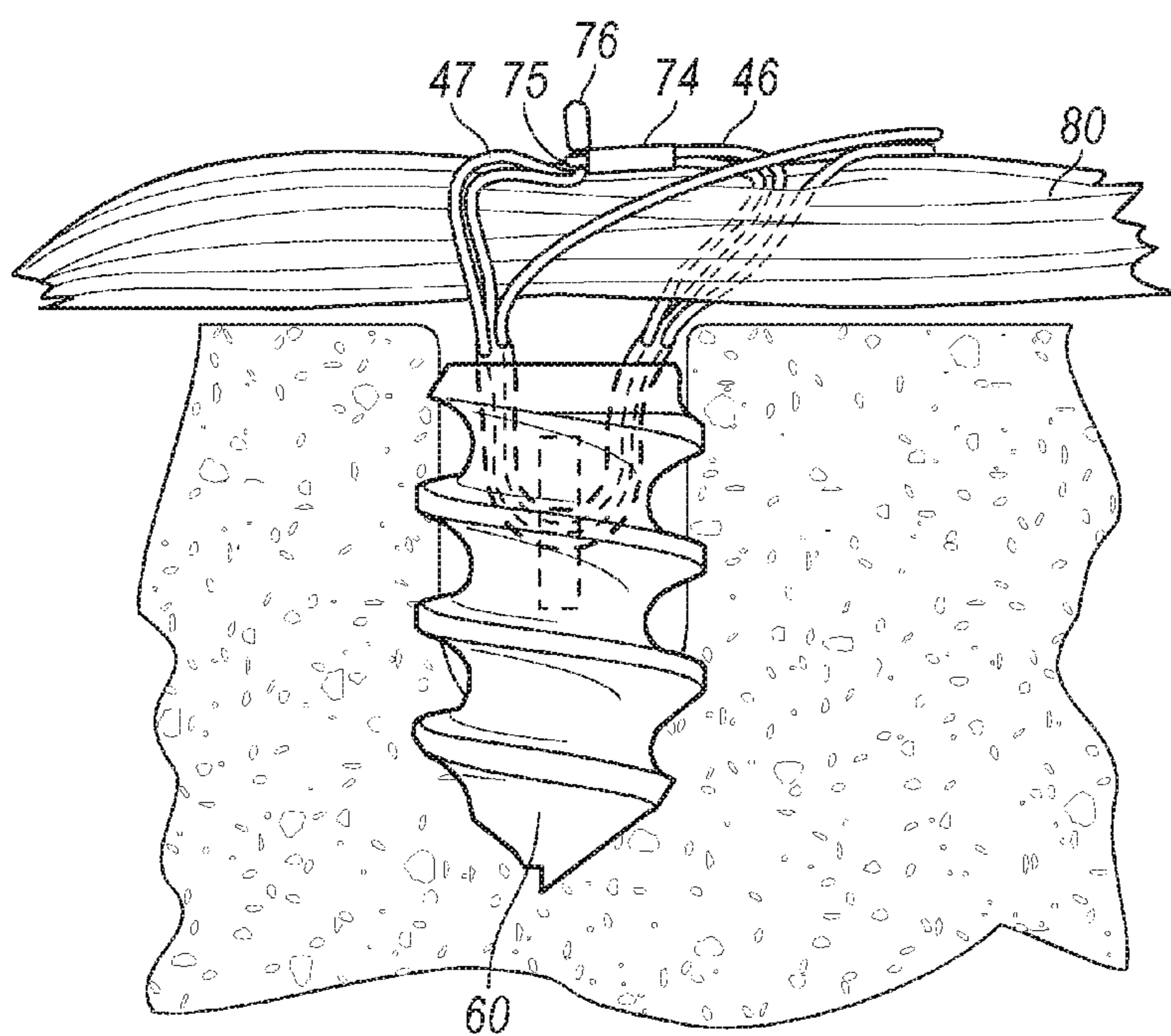
FIG. 16D
