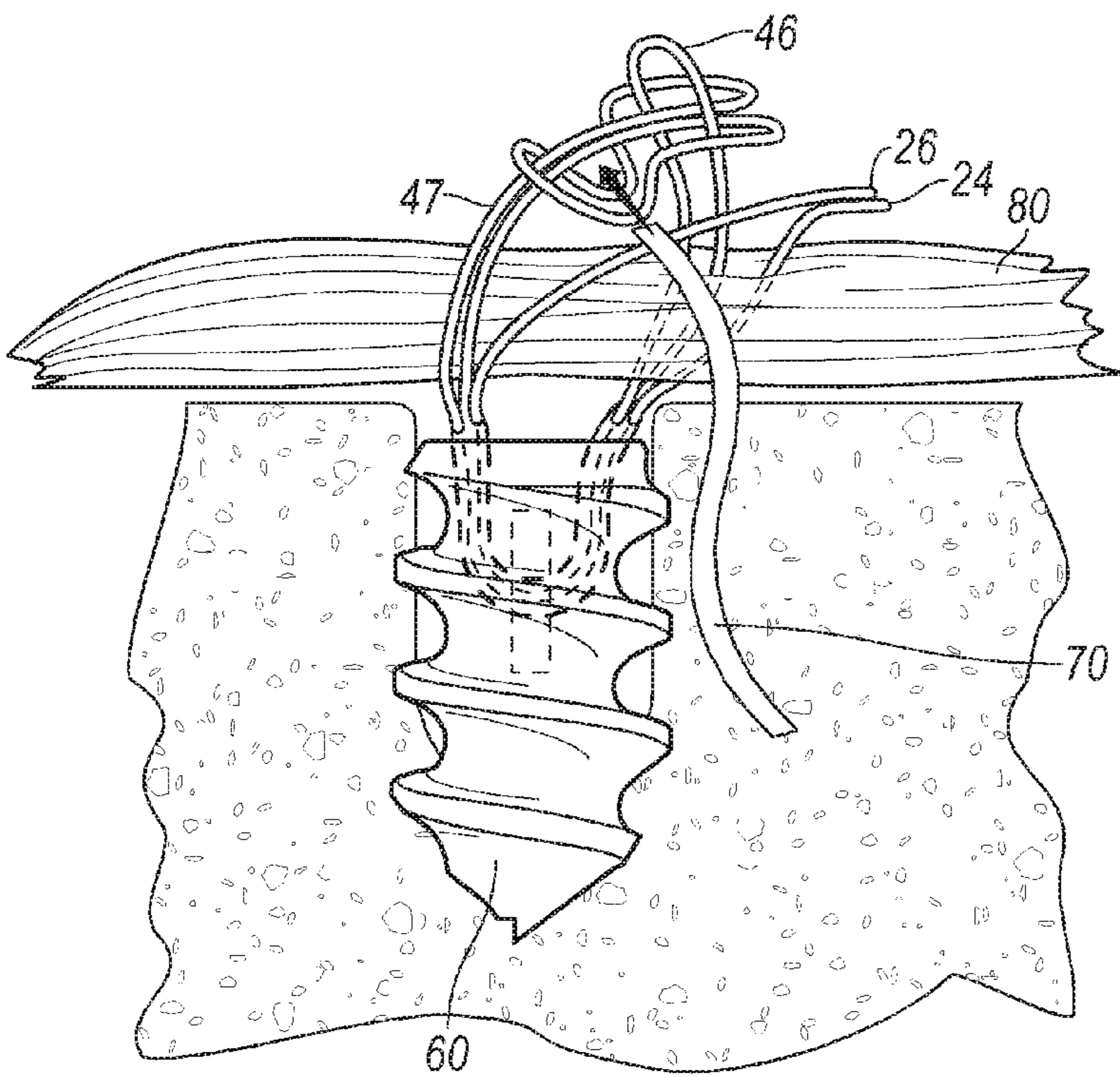
FIG. 17D
