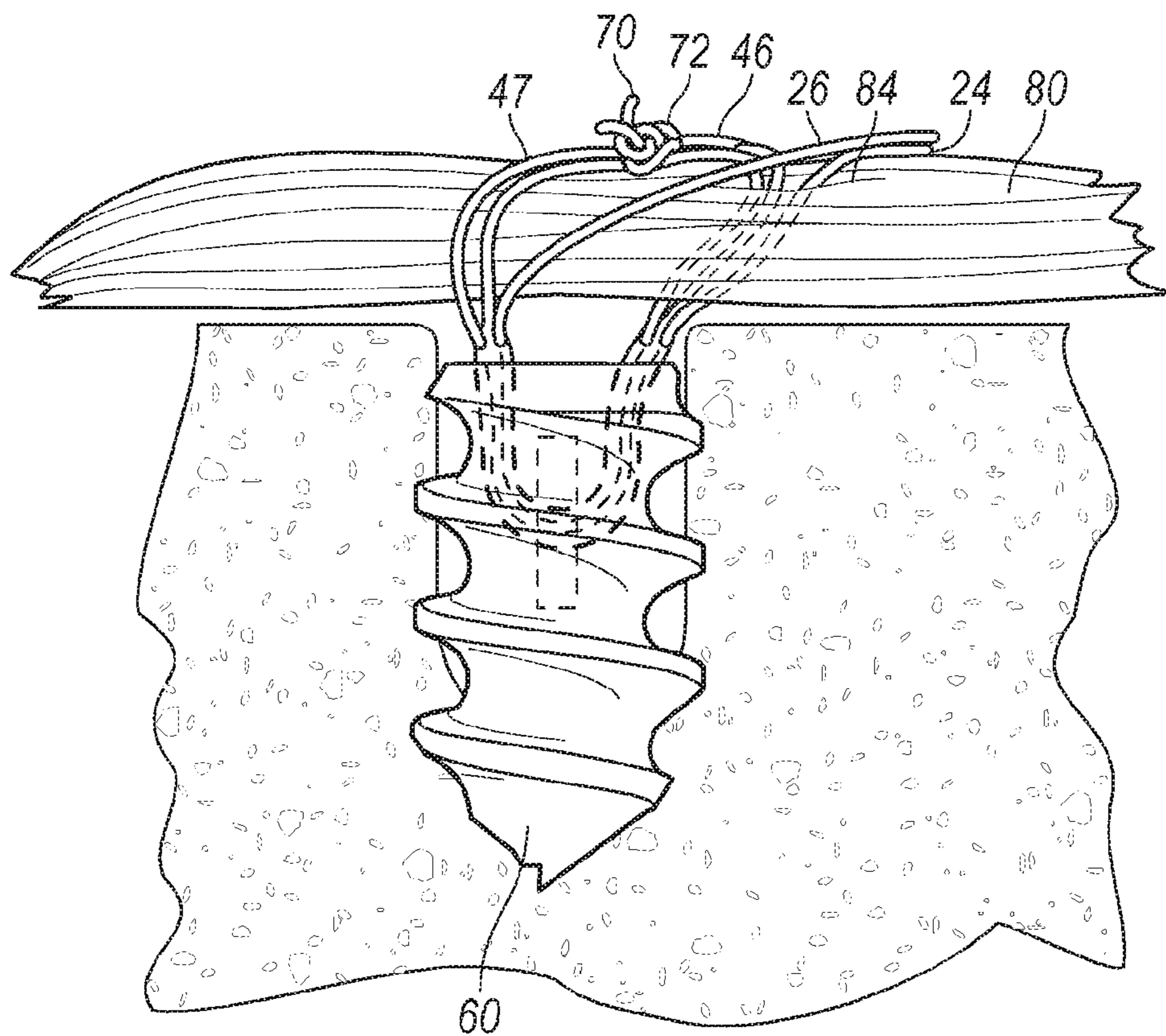
FIG. 15G
