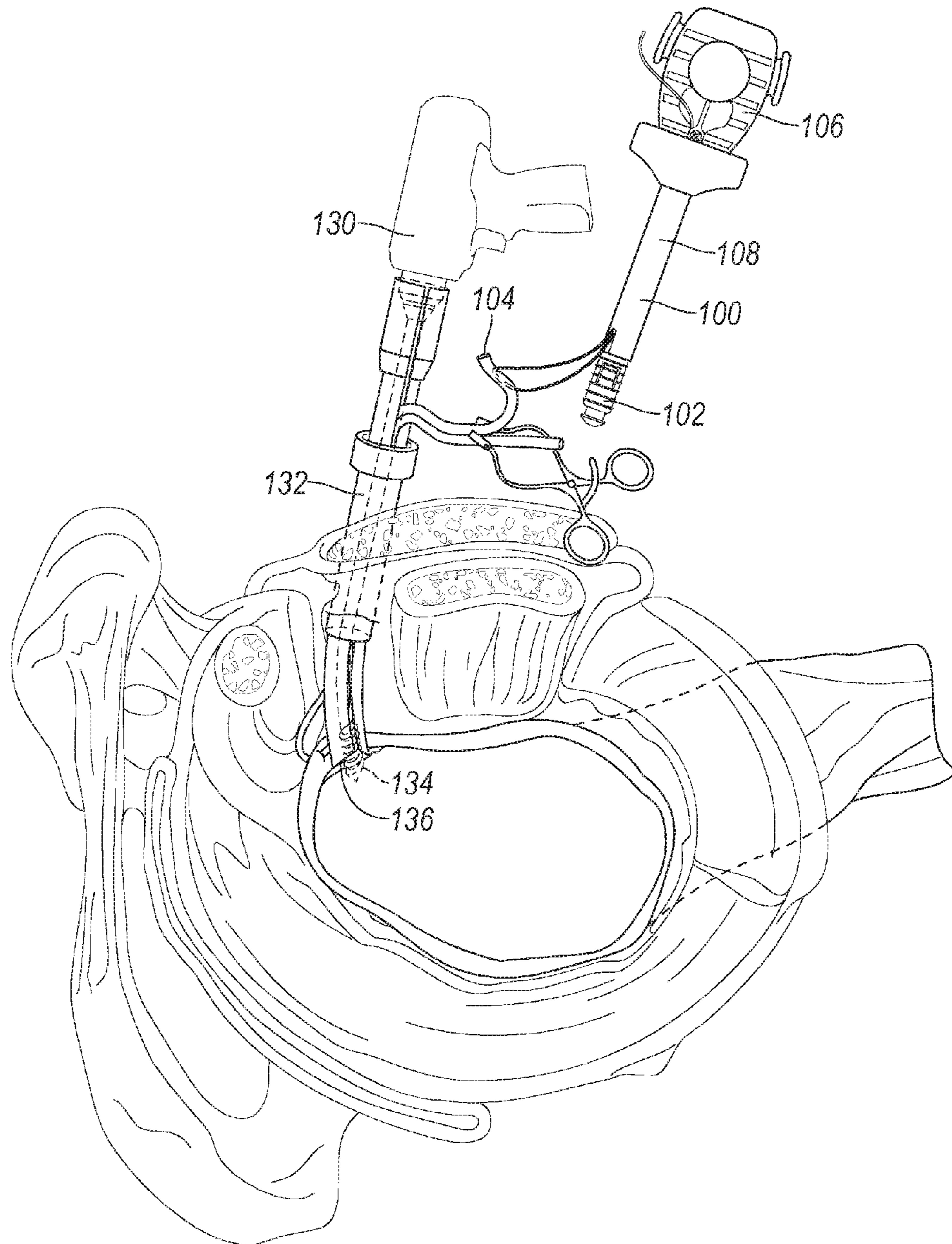
FIG. 26
