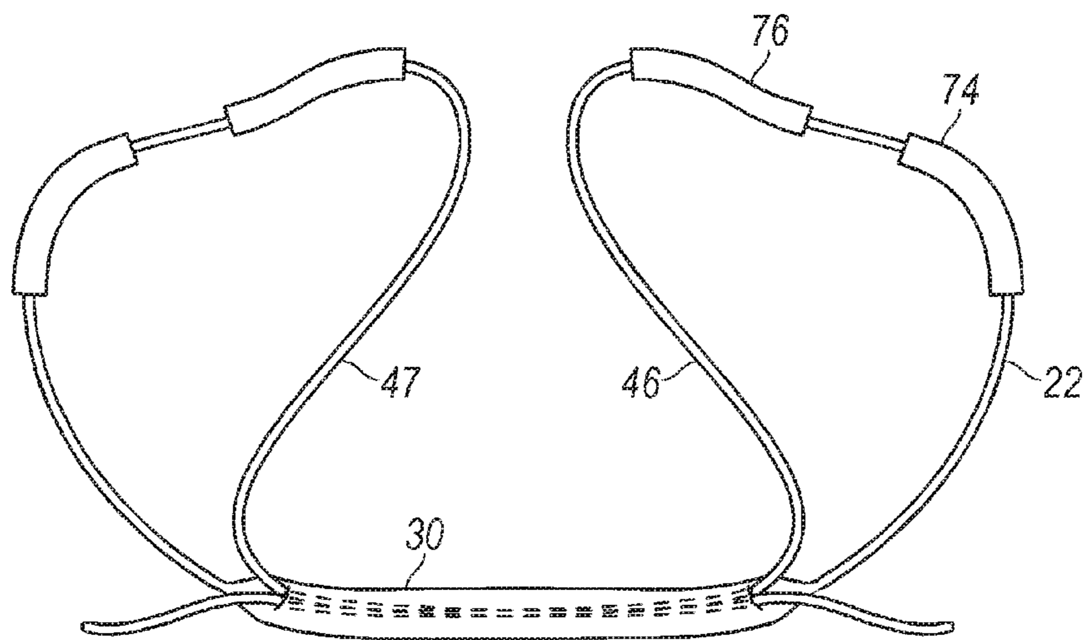
FIG. 18B
