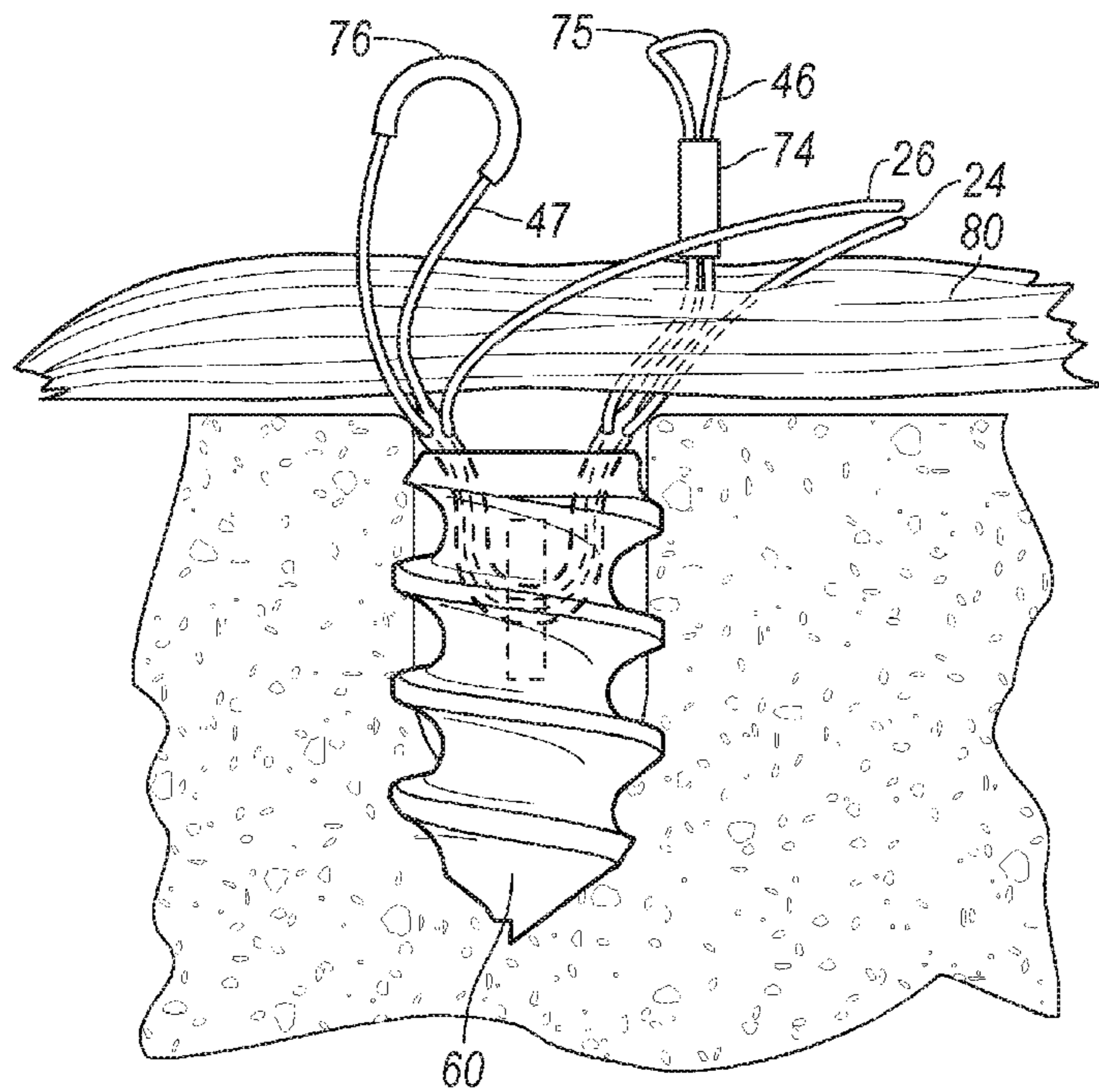
FIG. 16A
