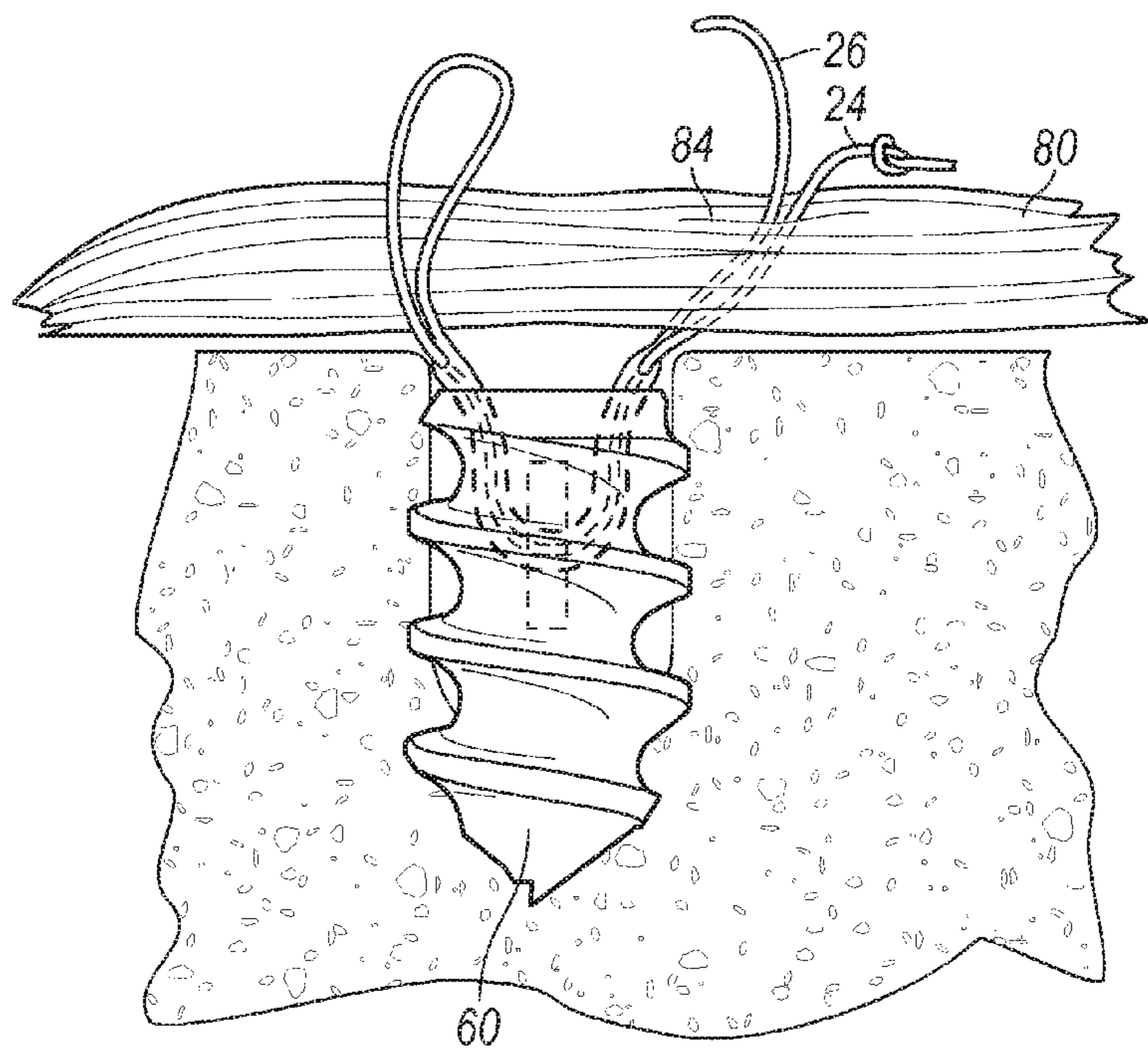
FIG. 15B
