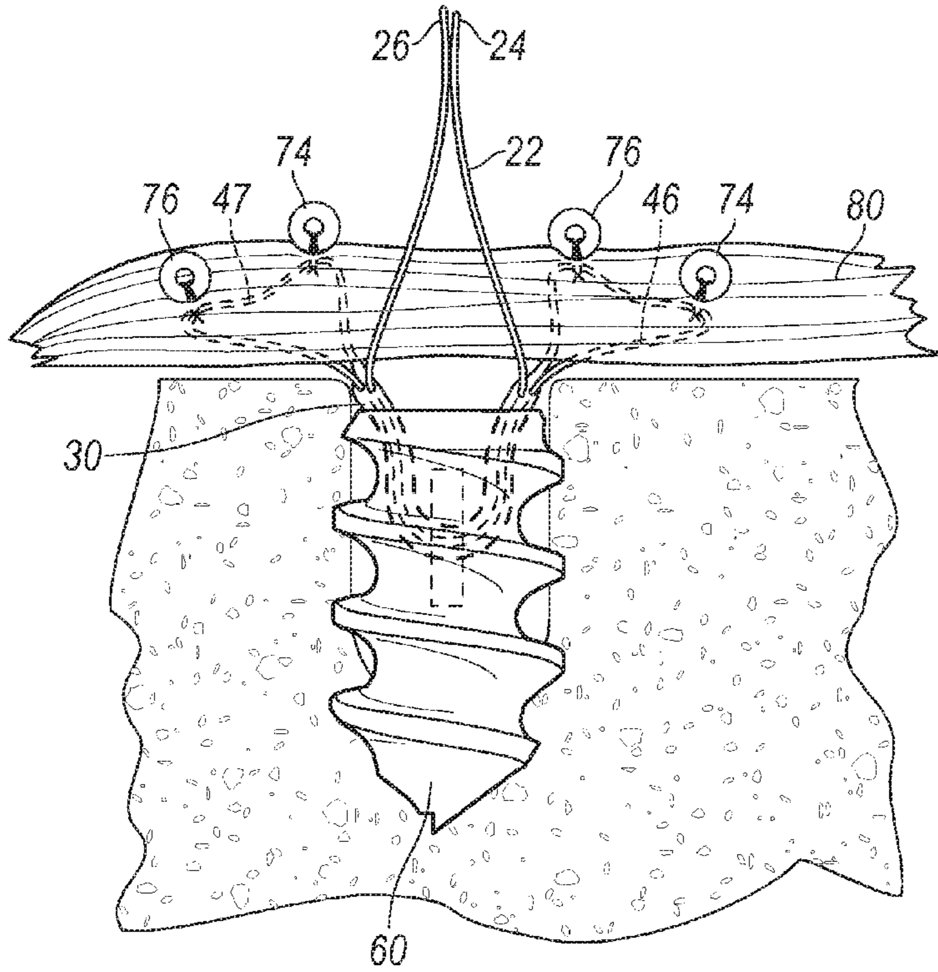
FIG. 18C
