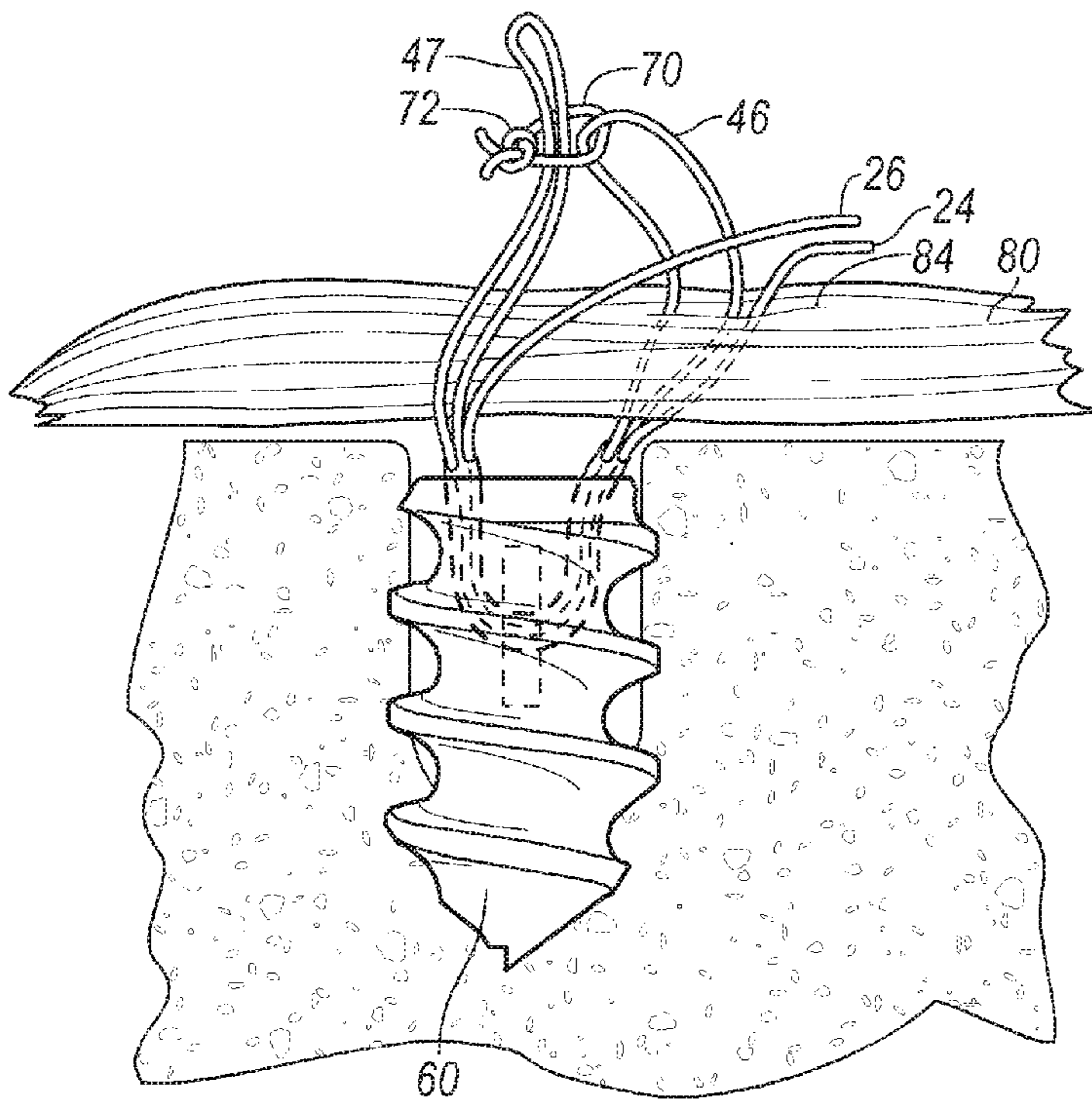
FIG. 15D
