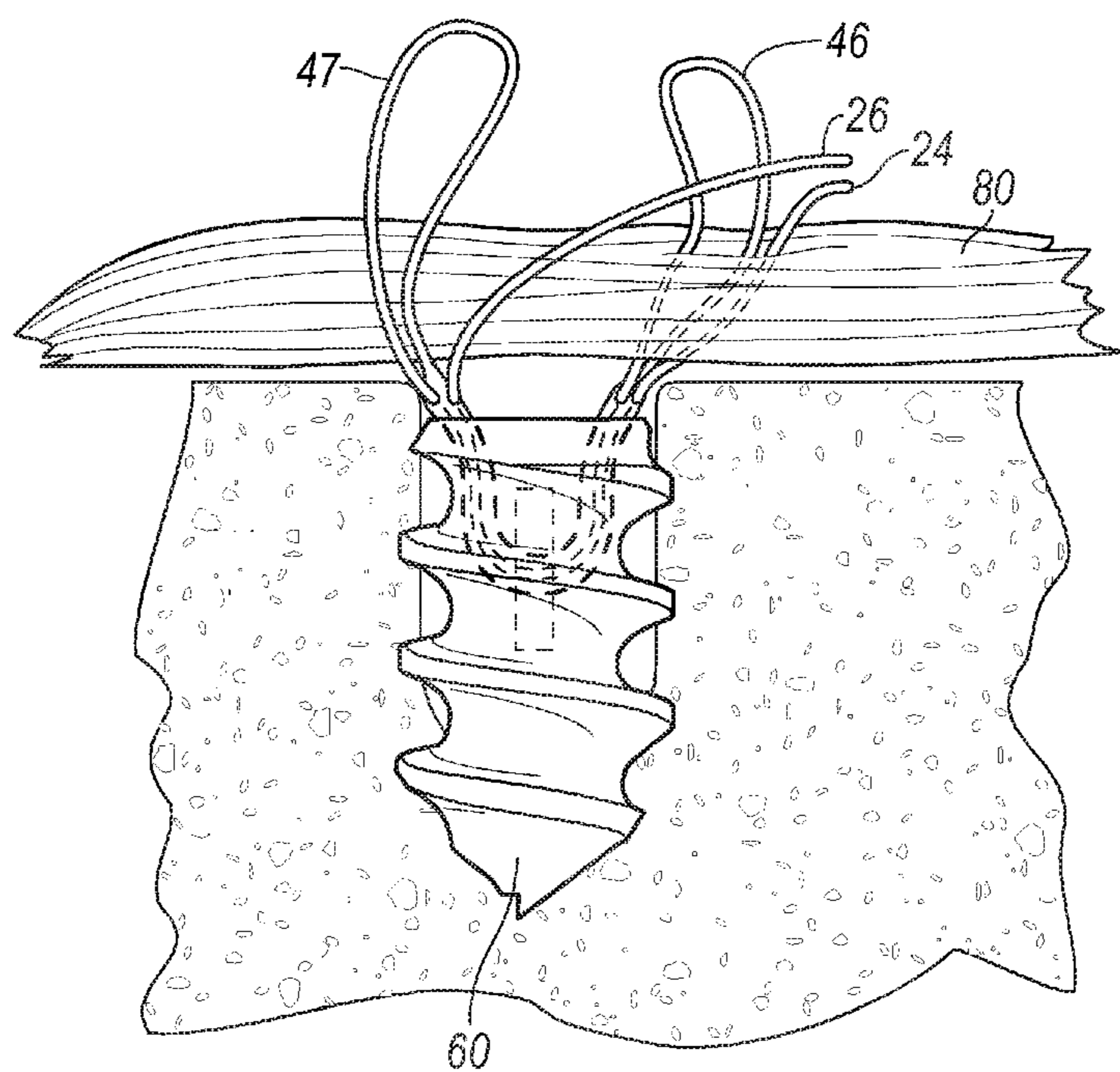
FIG. 17A
