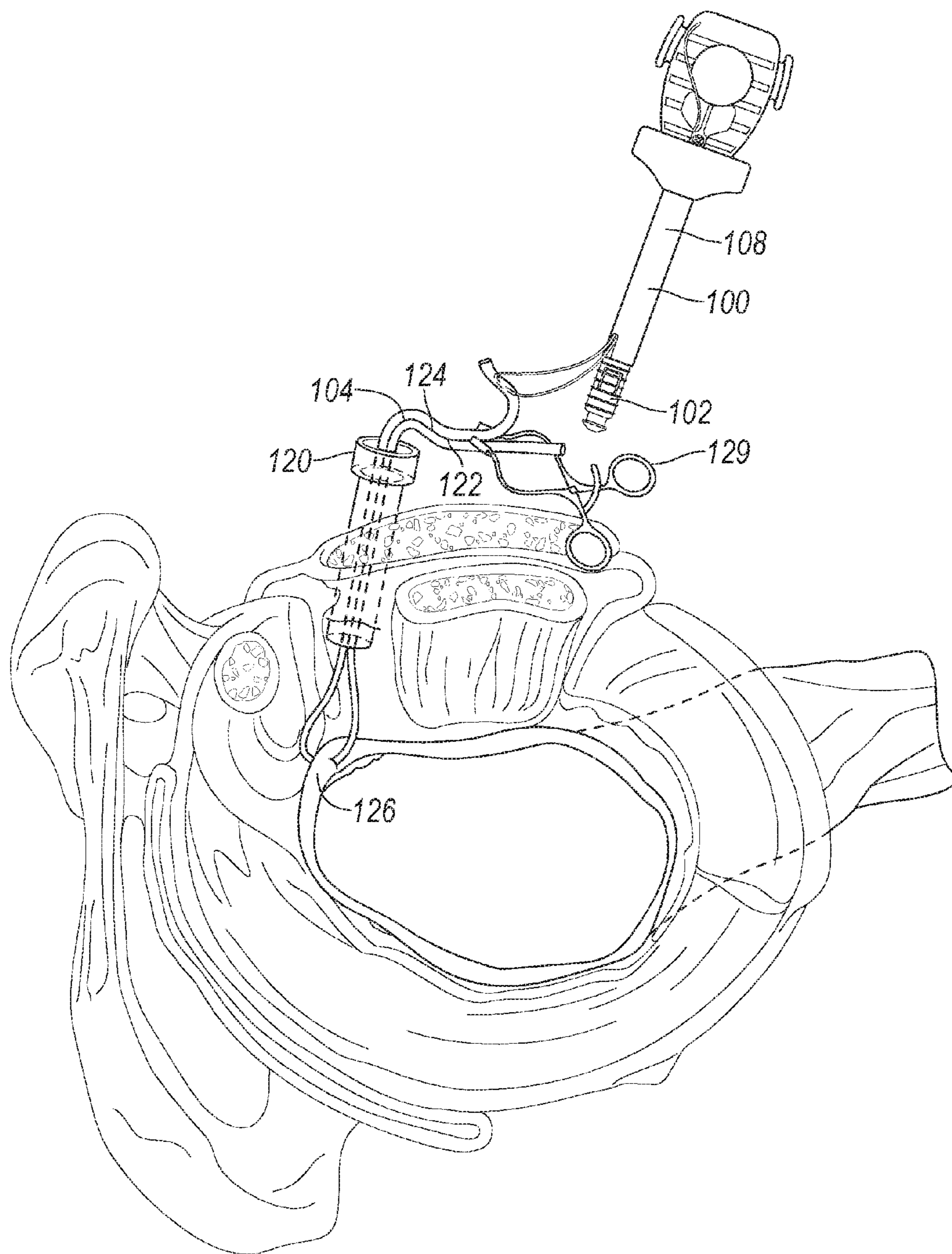
FIG. 24
