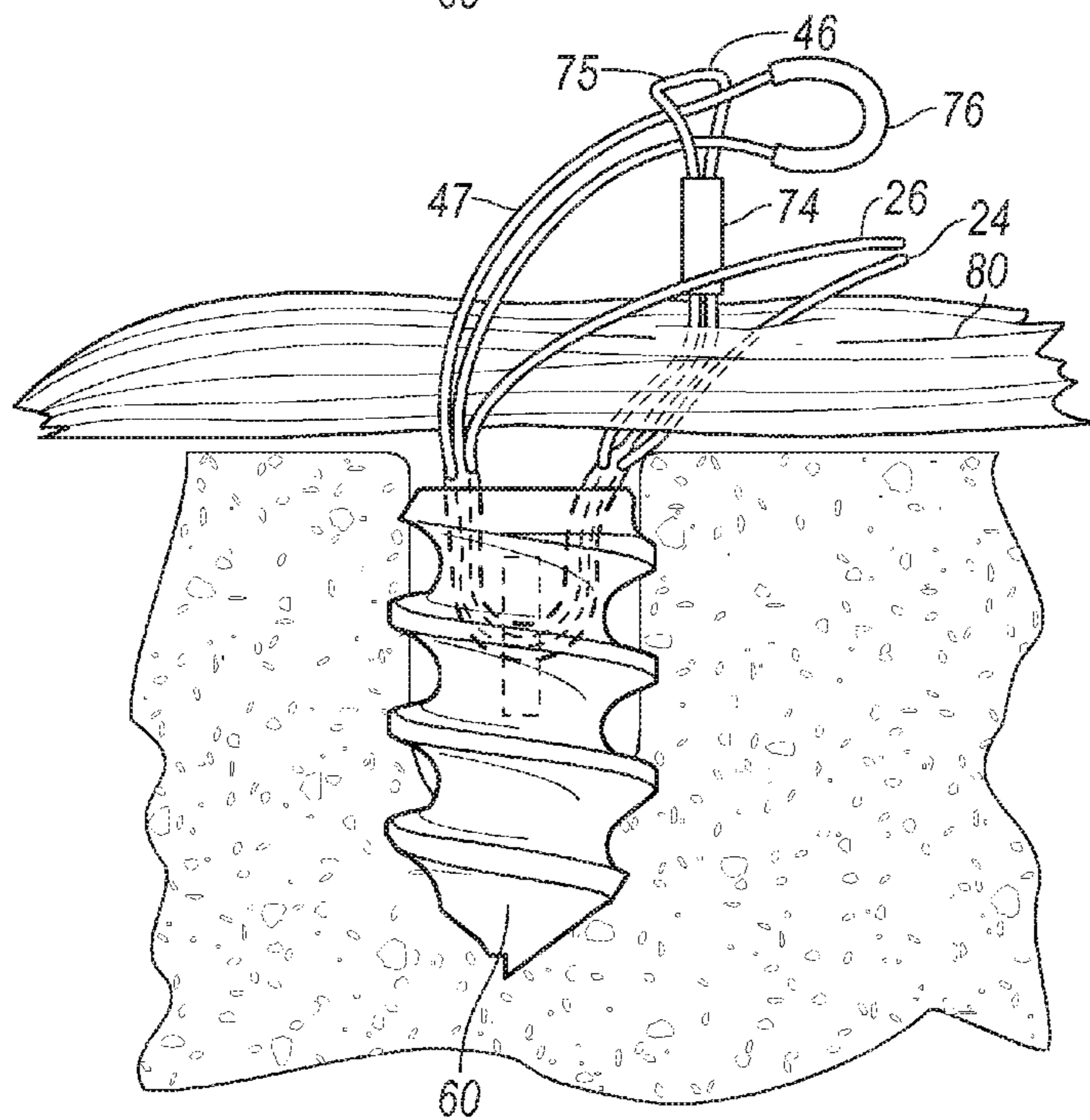
FIG. 16B
